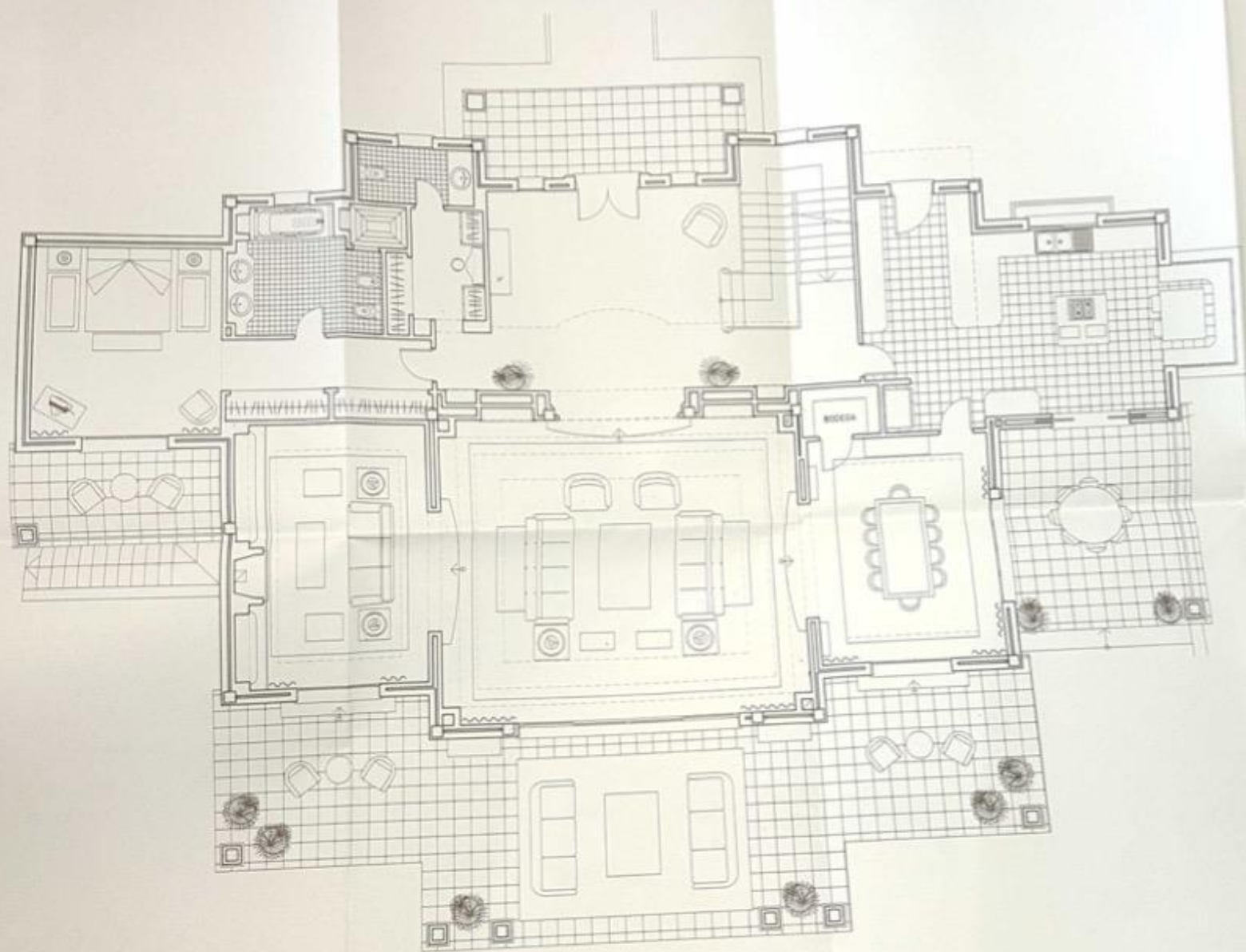
PLANTA BAJA
