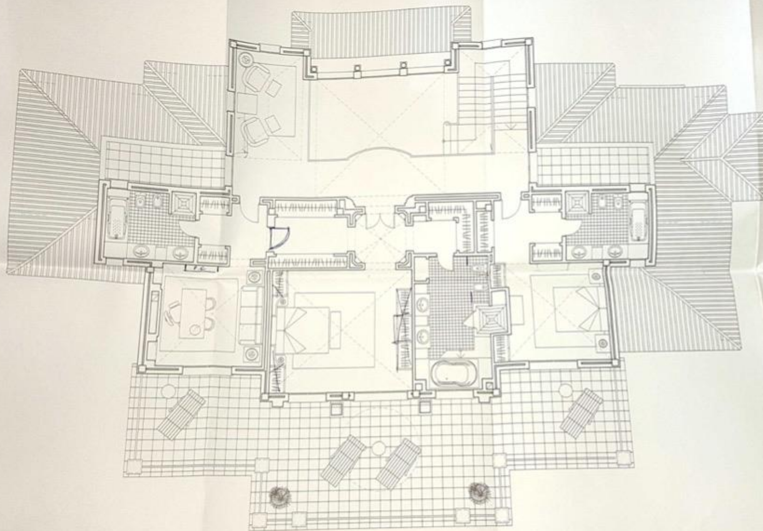
PLANTA ALTA
